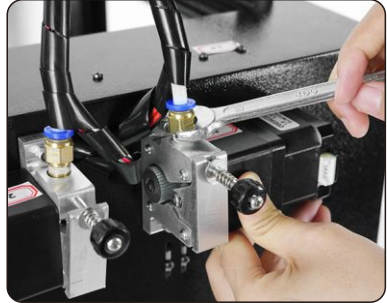
安装导管
